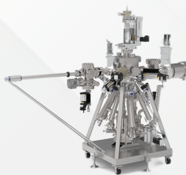
MBE СИСТЕМЫ
